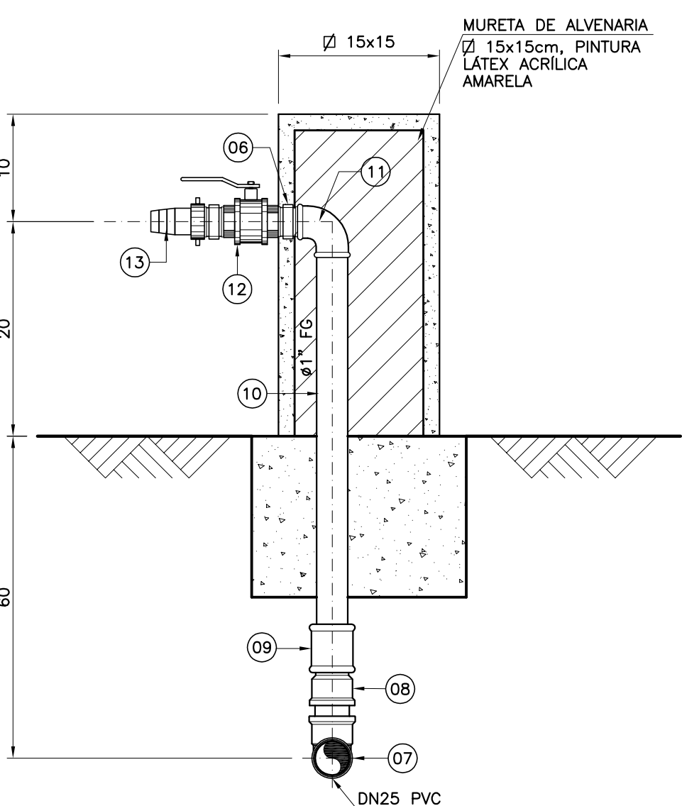
DETALHE 1 PONTO DE ÁGUA DE SERVIÇO (PAS) S/ESCALA
