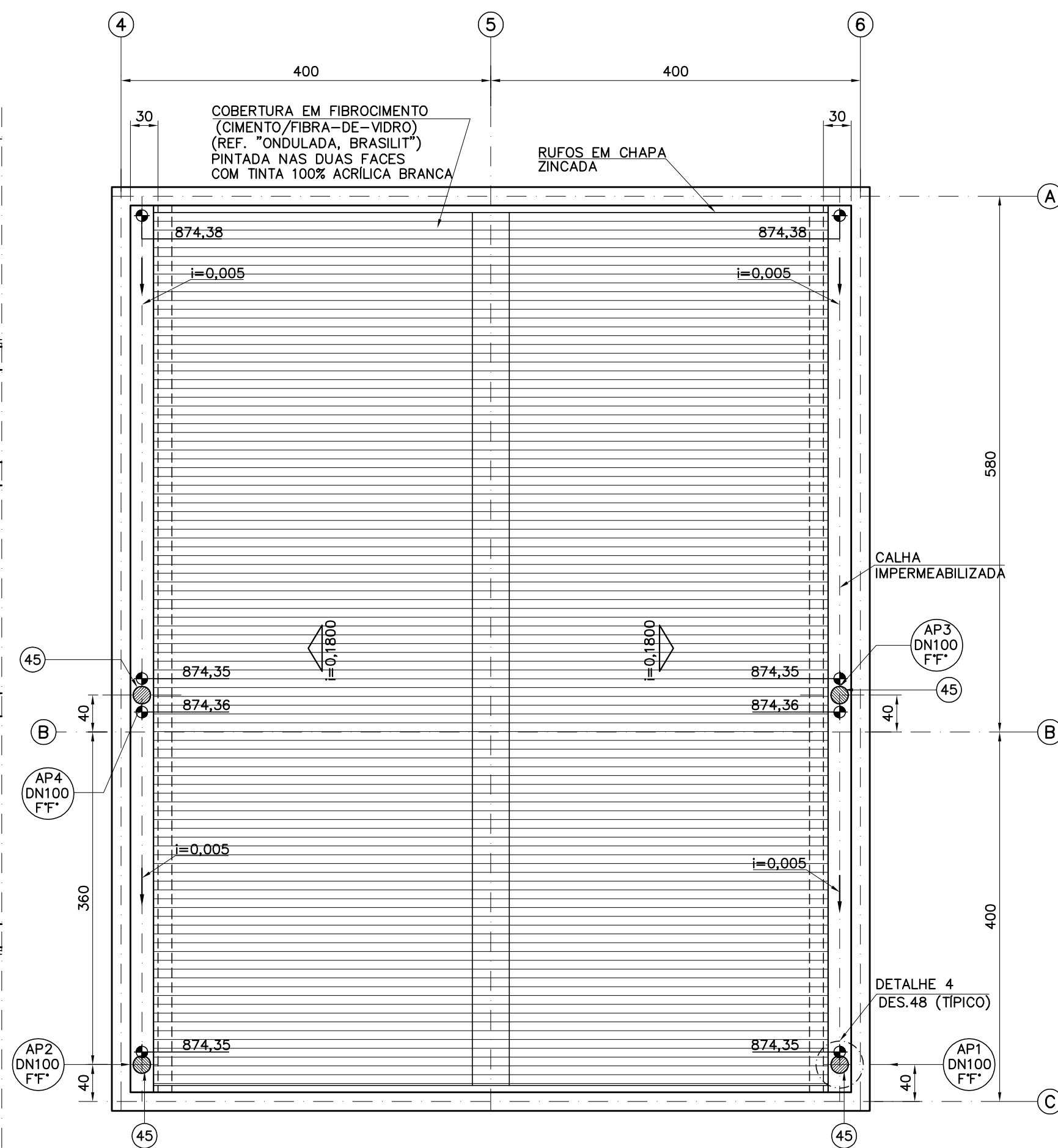
PLANTA DE COBERTURA ESC. 1:50
