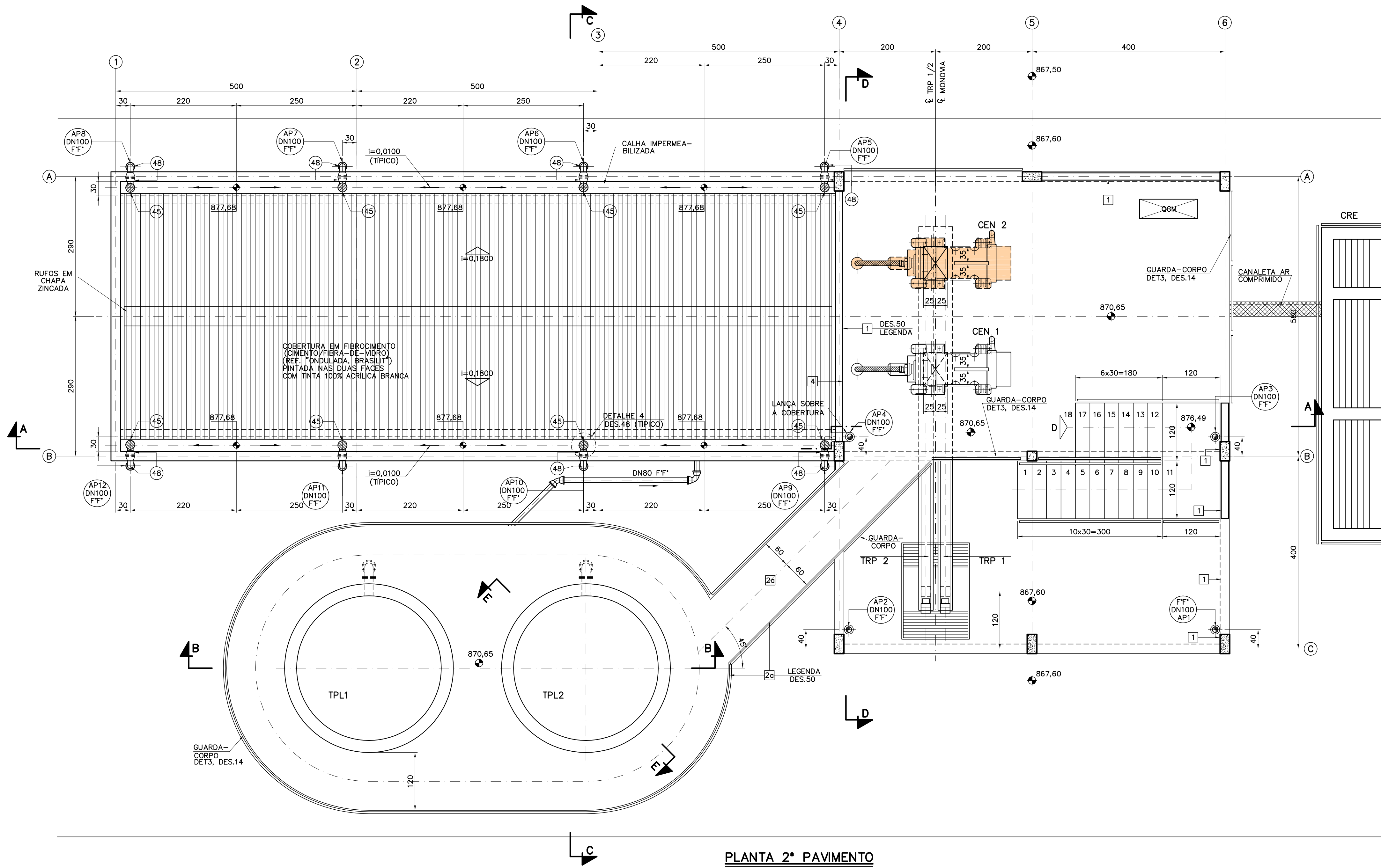
PLANTA 2º PAVIMENTO ESC. 1:50
